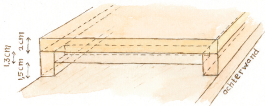
detail invliegopening
