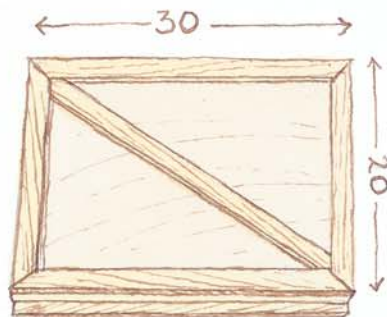
detail rechterluik
