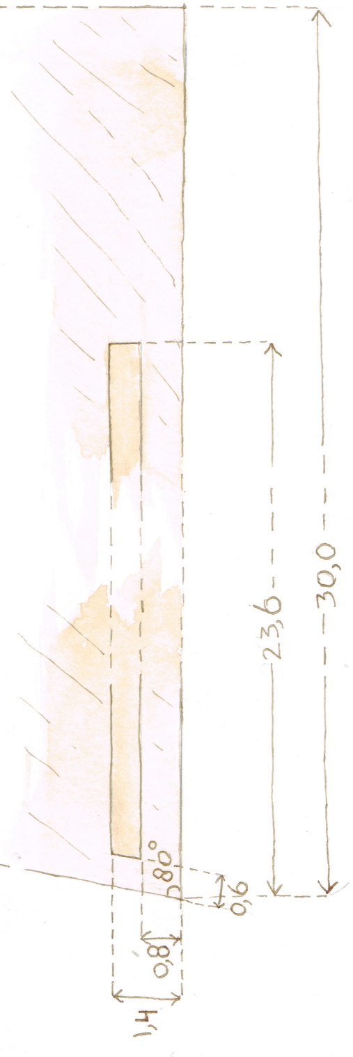
binnenkant zijwand E: sleuf detail
