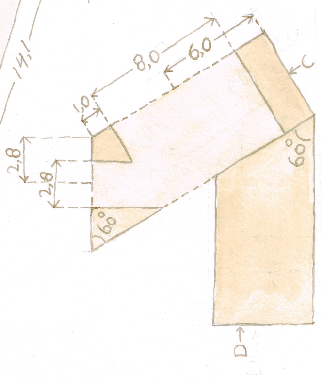
zaagpositie Cen D dwarsdoorsnede boormal
