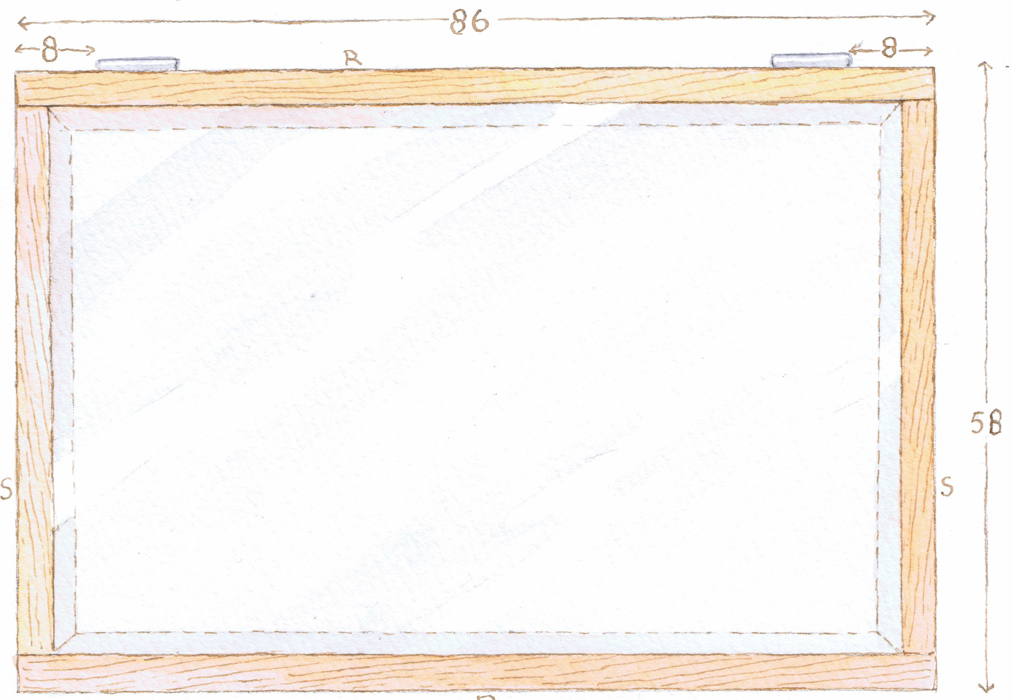
onderkant deksel
